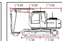
＜クローラ車両＞
