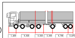
＜フルトレーラ＞
