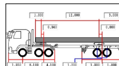
＜ポールトレーラ＞
