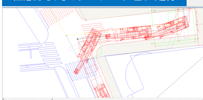
任意形状でのアニメーション走行
