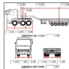
＜セミトレーラ＞
