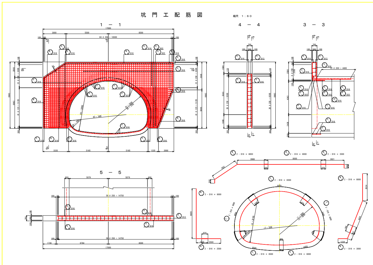
坑門工配筋図
